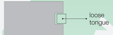
Рисунок 6 (справа). Пример усиления проёмов деревянным гребнем.
