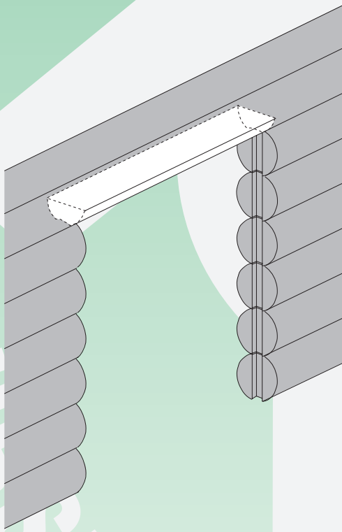
Рисунок 5 (слева). Дверной и оконный проём. Пропилы указанных проёмов можно делать по месту.
